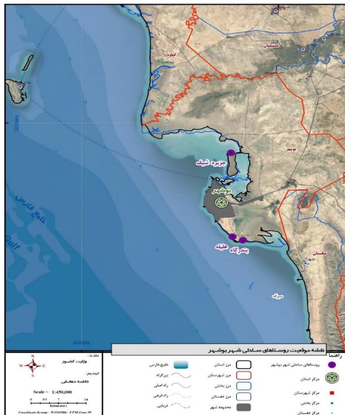
شکل ۴. موقعیت روستاهای ساحلی شهر بوشهر
